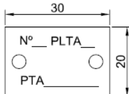
Figura 22. Identificación fusibles.
